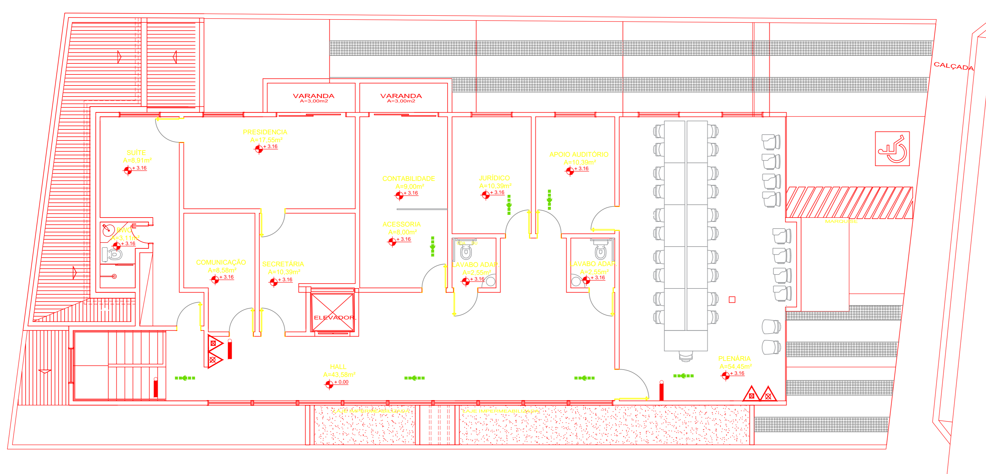
PLANTA BAIXA PAVT. SUPERIOR ESCALA 1/75
